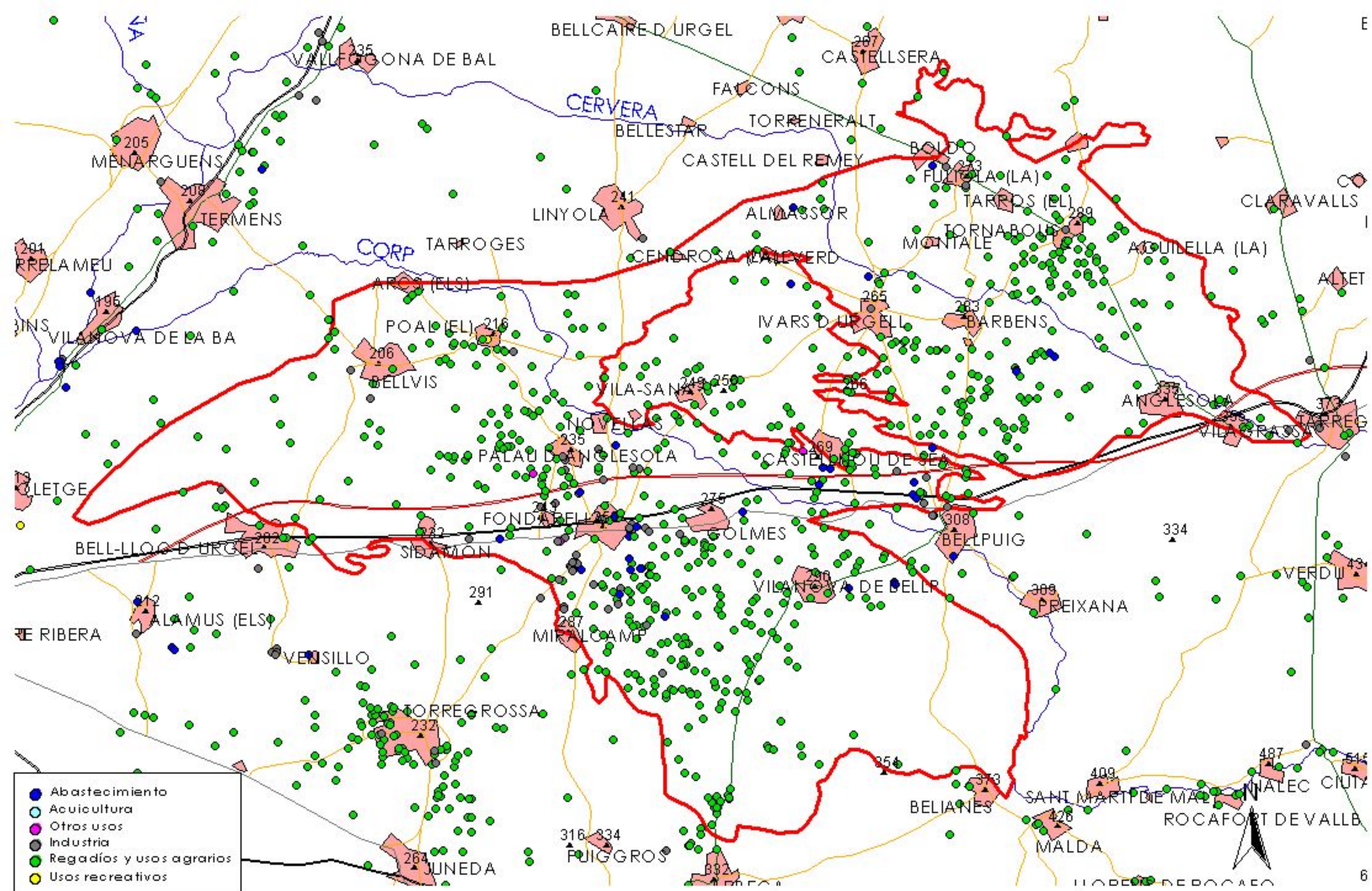
MAPA 9.1: MAPA DE EXPLOTACIÓN DE AGUAS SUBTERRÁNEAS 90_063 ALUVIAL DE URGELL
