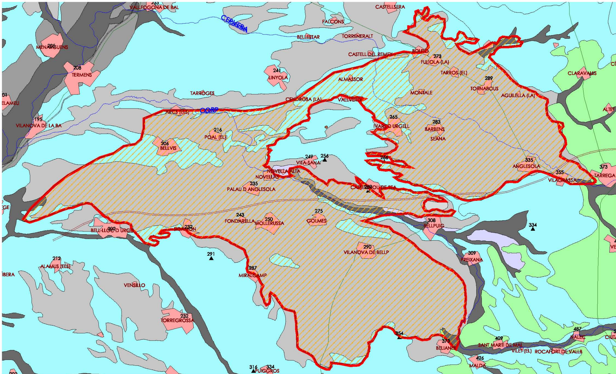
MAPA 7.1: MAPA DE ÀREAS DE RECARGA 90_063 ALUVIAL DE URGELL
