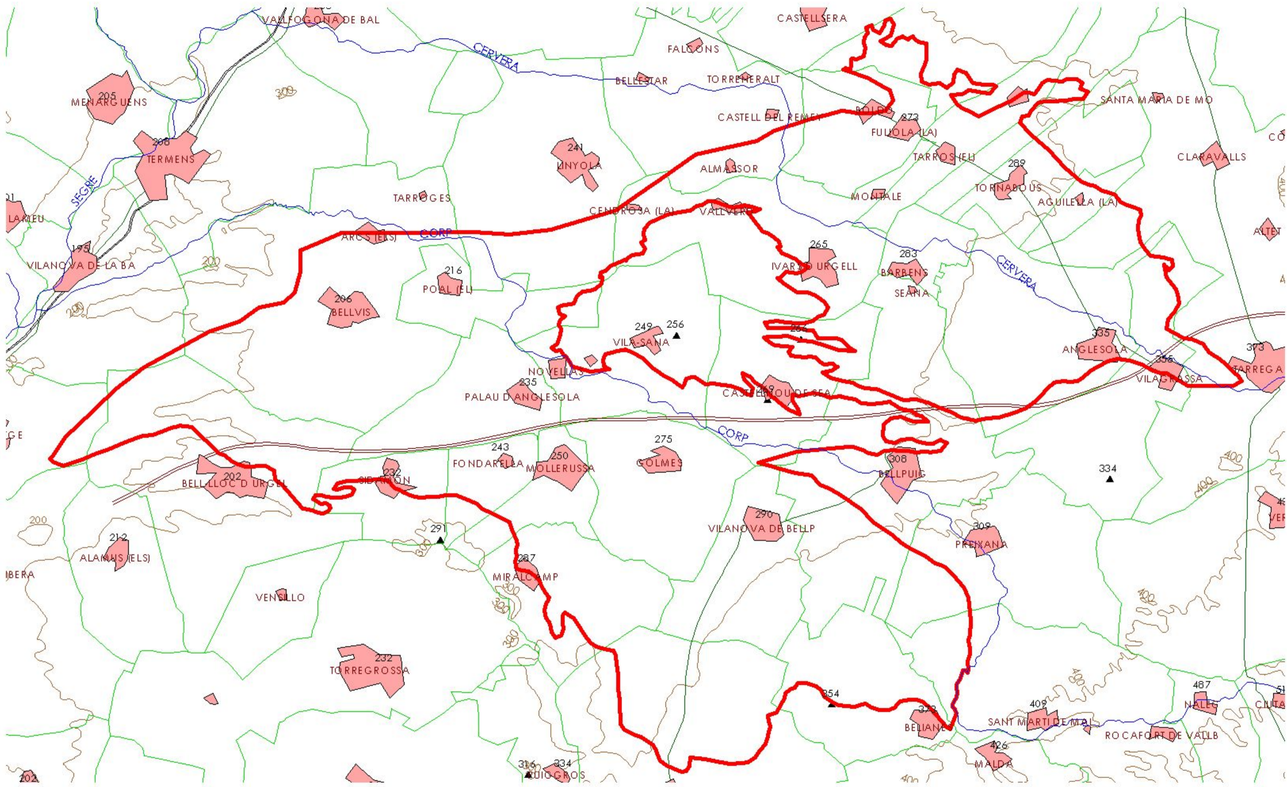
MAPA 1.1: MAPA DE IDENTIFICACIÓN 90_063 ALUVIAL DE URGELL
