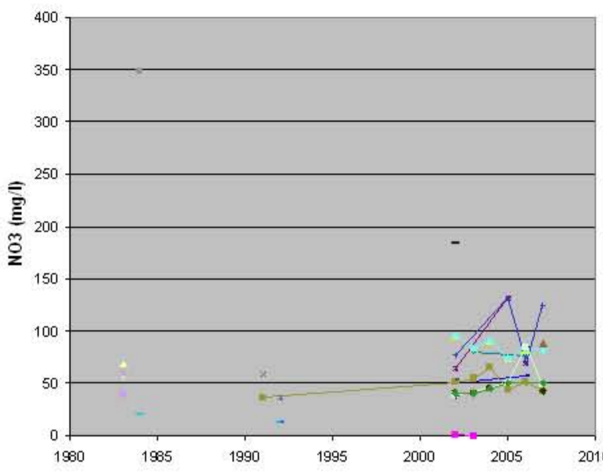
Evolución Temporal de Nitrato de la masa 90_063
