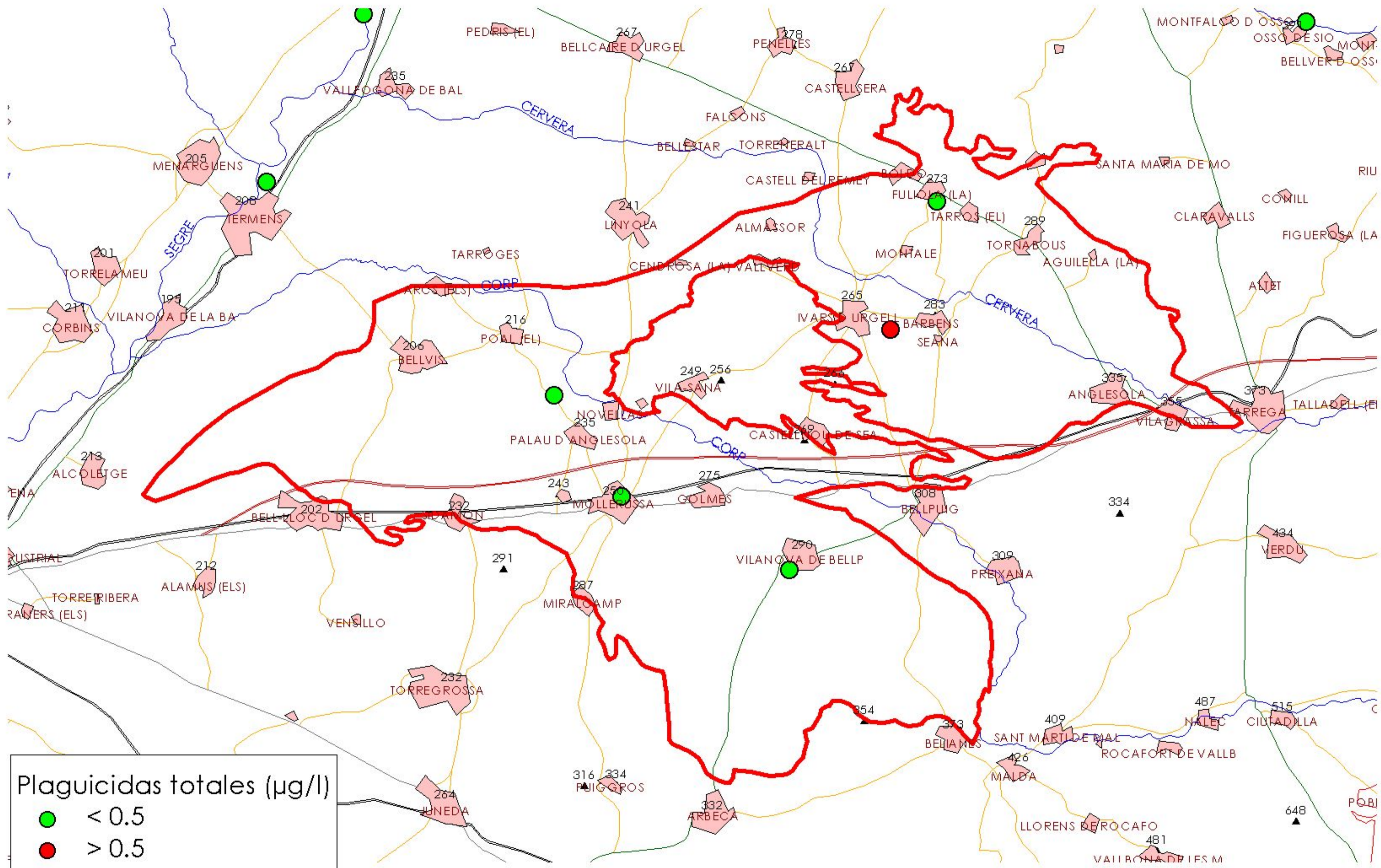
MAPA 10.6.2: MAPA DE NIVELES DE REFERENCIA 90_063 ALUVIAL DE URGELL
