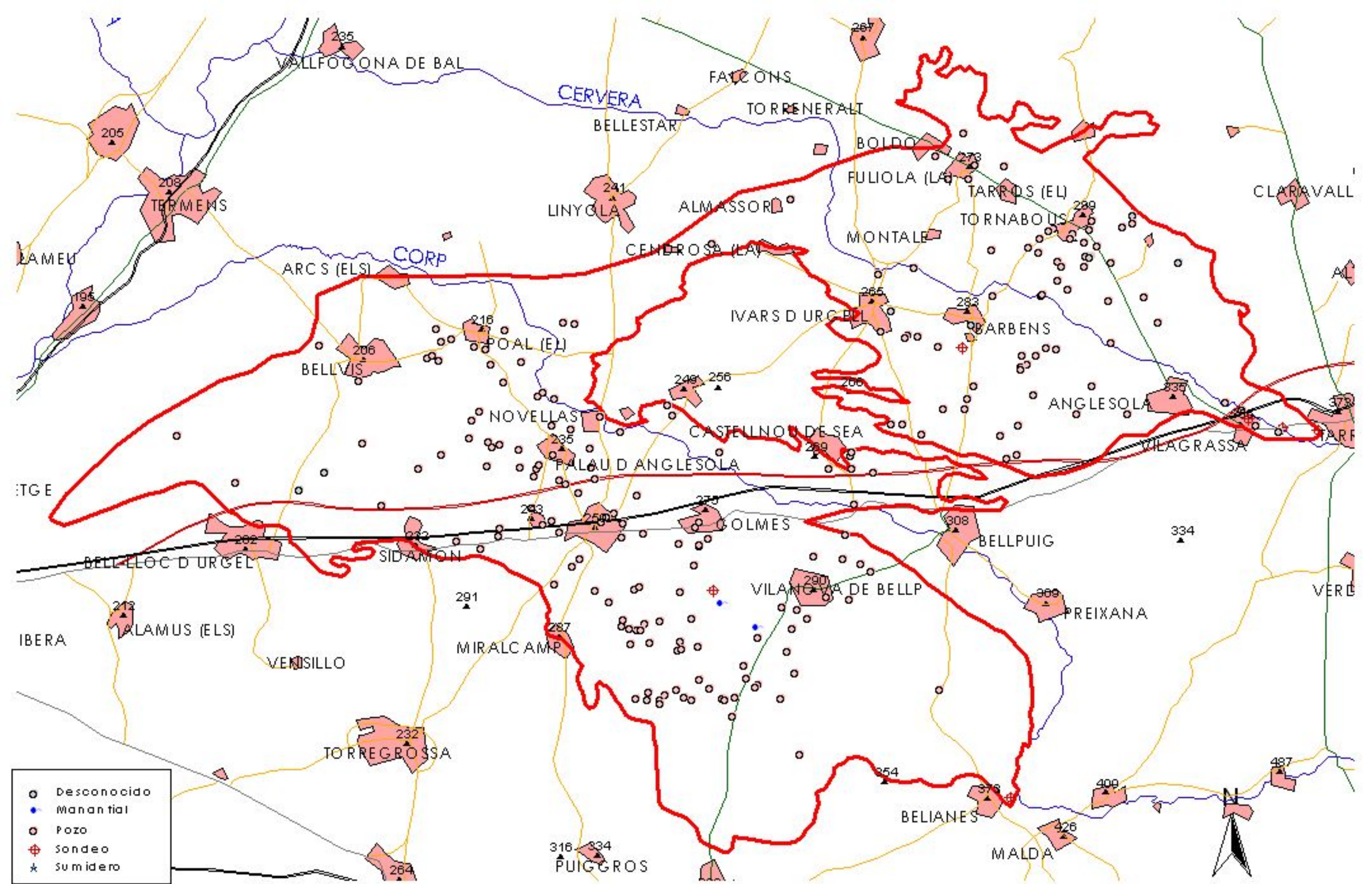
MAPA 9.2: MAPA DE INVENTARIO DE PUNTOS DE AGUA 90_063 ALUVIAL DE URGELL
