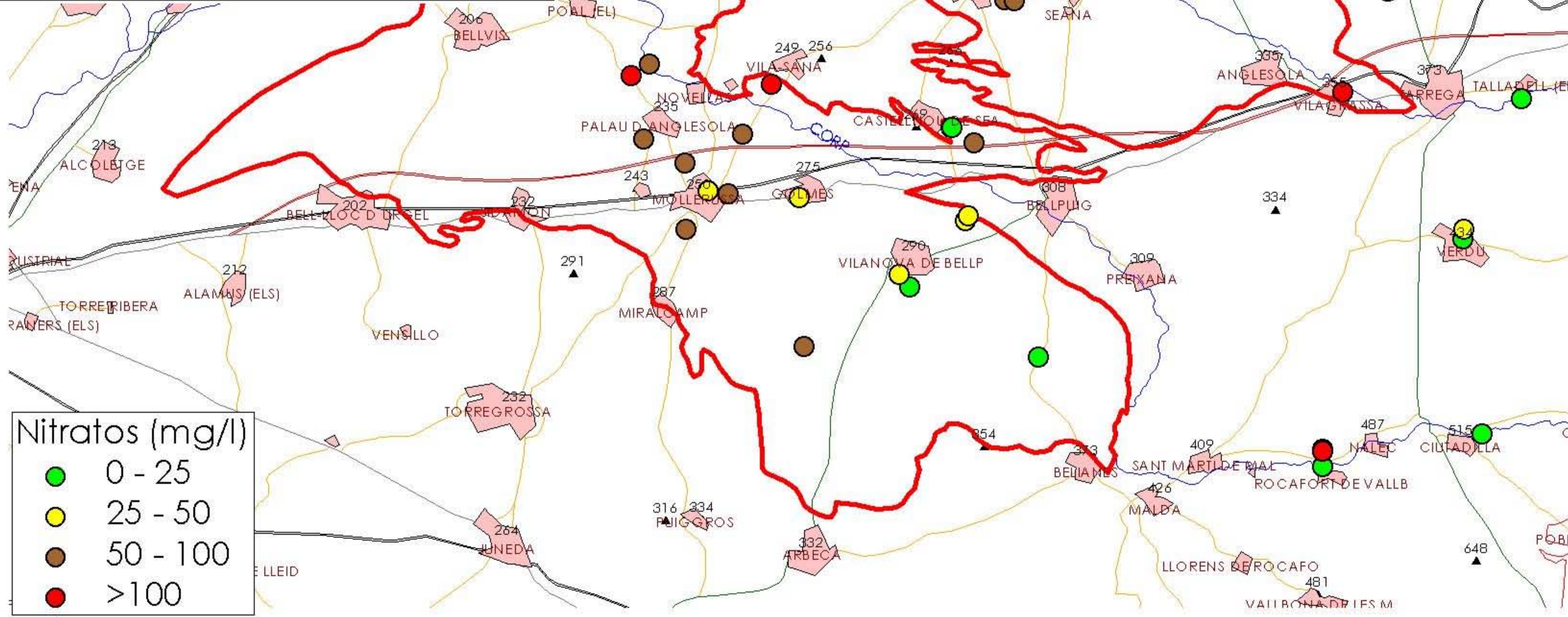
MAPA 10.3.1: MAPA DE NIVELES DE REFERENCIA 90_063 ALUVIAL DE URGELL
