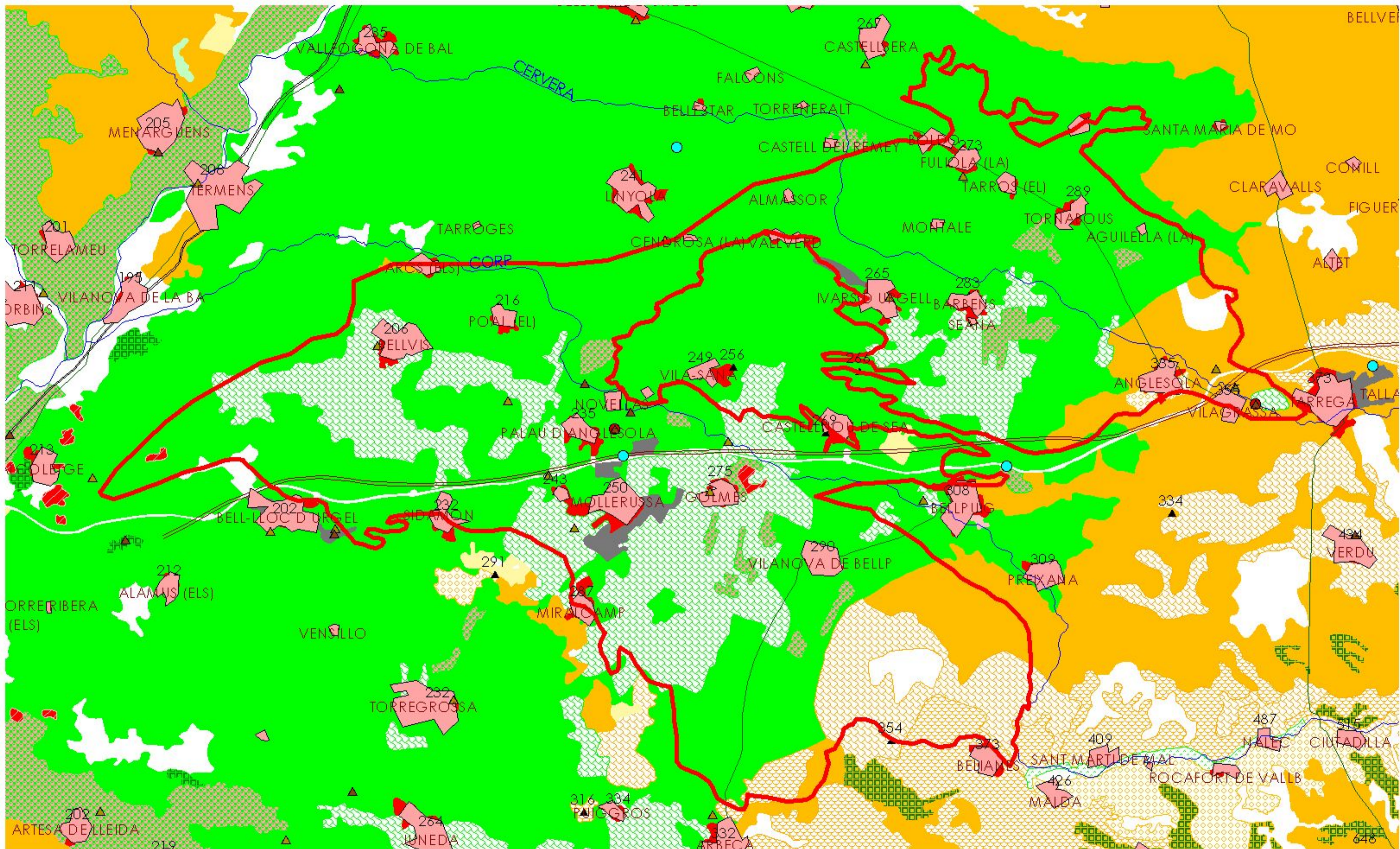
MAPA 14.1: MAPA DE SITUACI6N DE ACTIVIDADES CONTAMINANTES 90_063 ALUVIAL DE URGELL
