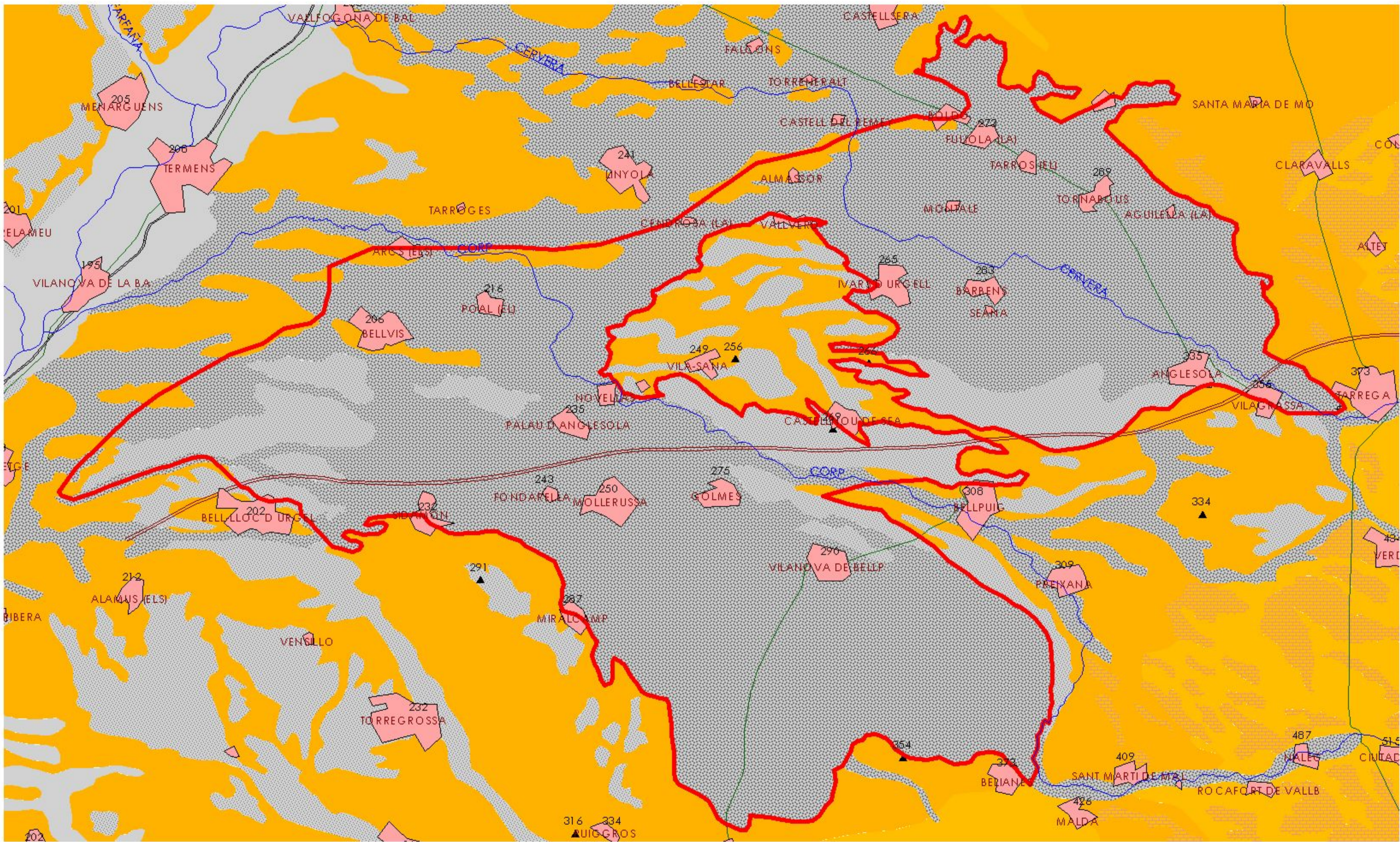
MAPA 2.1: MAPA GEOLÓGICO 90_063 ALUVIAL DE URGELL
